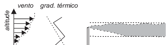
Condição LIMITADA - inversão térmica Pluma entre duas camadas de inversão ou condição neutra um levemente instável ou estável abaixo da inversão.
