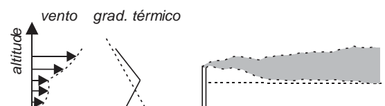
Condição ANTIFUMIGANTE - inversão térmica A pluma possui energia suficiente para atravessar a capa de inversão. A parte inferior da pluma fica aprisionada na parte superior da inversão. A parte superior da pluma amplia a difusão. Melhor caso de dispersão de plumas (chaminés altas).
