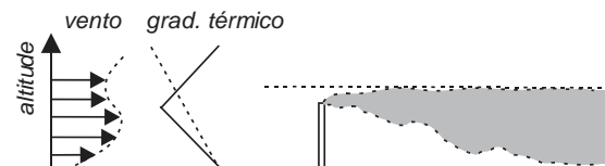
Condição FUMIGANTE - instabilidade+inversão térmica A pluma fica aprisionada em capa de inversão térmica que se rompe pela parte inferior (instável). Altas concentrações de poluentes (risco).
