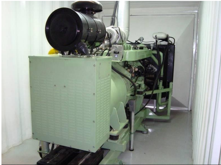
Figura 52 – Motor ciclo Otto adaptado a biogás. Fonte: CENBIO, 2009.
