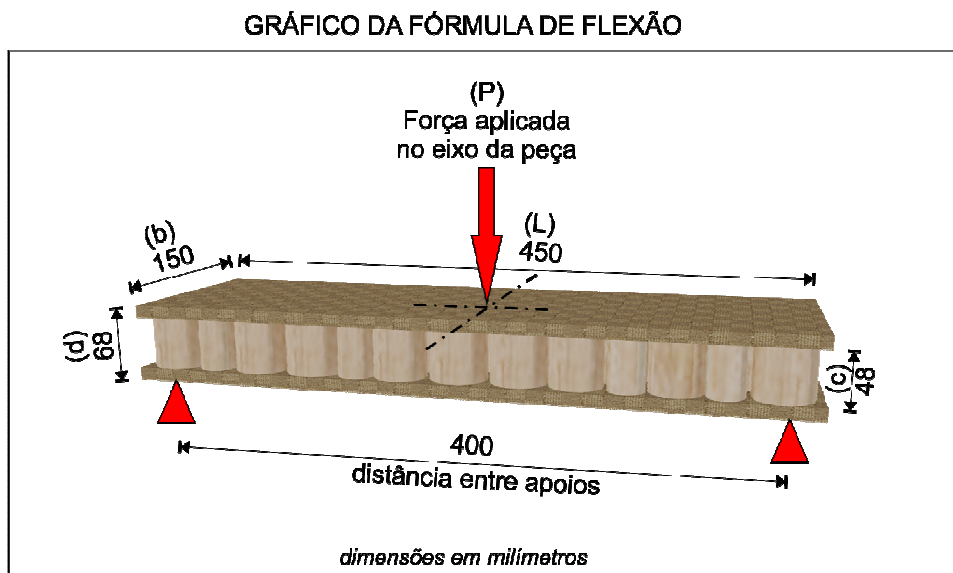
Figura 110: Exemplo do carregamento no ponto central e esquema (ASTM C 393-00)
