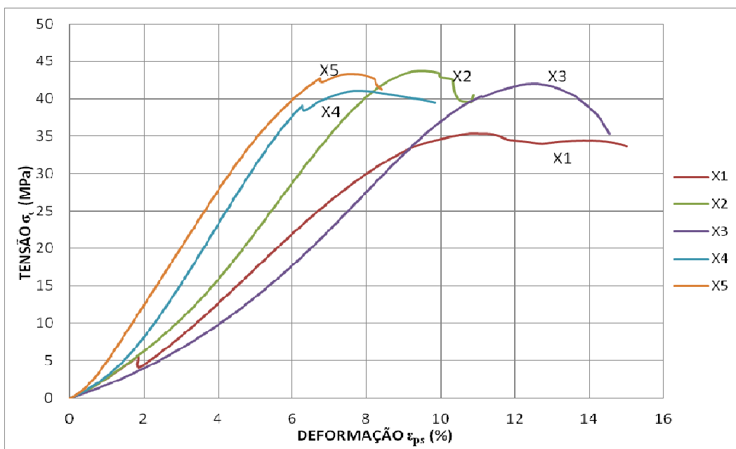
Figura 134: Tensão de compressão ( \sigma ) vs. deformação do painel sanduíche de bambu ( \epsilon_{ps} ).vs.
