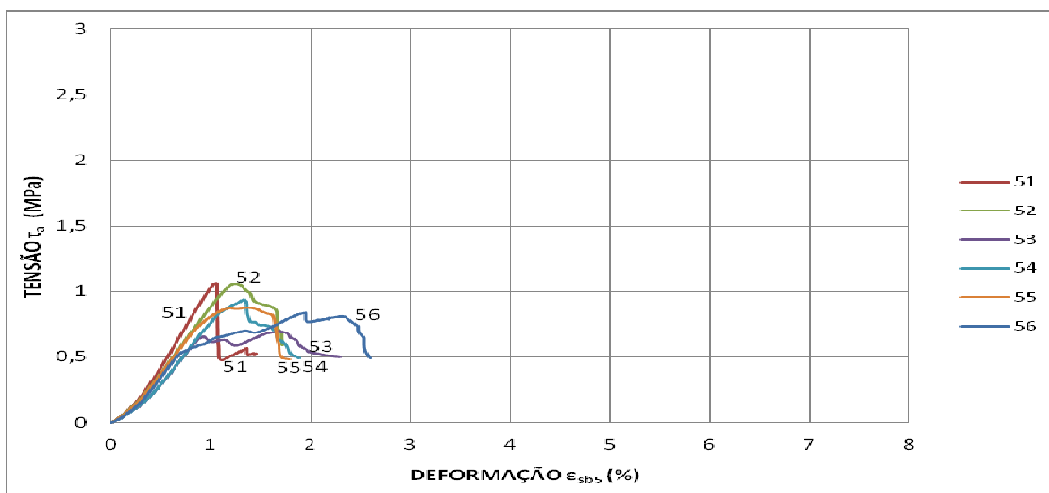
Figura 144: Tensão de cisalhamento do adesivo ( \tau_a ) vs. deformação dos corpos de prova ESB5 ( \epsilon_{sb5} ).
