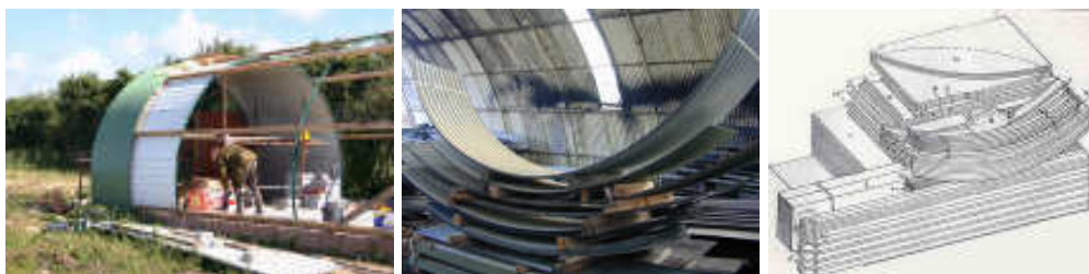
Figura 35: Abrigo nissen. A) e B) Montagem (Fonte: Langham, 2012); C) Peças desmontadas (Fonte: News Domain, 2012)
