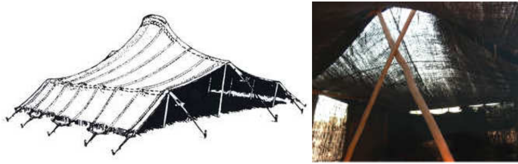
Figura 11: A) Cobertura estrutural tracionada; e B) Resfriamento passivo. (Fonte: Politecnico di Milano A) Autora: Francesca Focolari, 2008; B) Autor: T. Berger, 2005)
