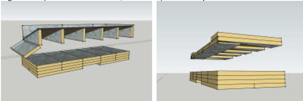
Figura 100: A) Desmontagem do telhado B) Abrigo desmontado
